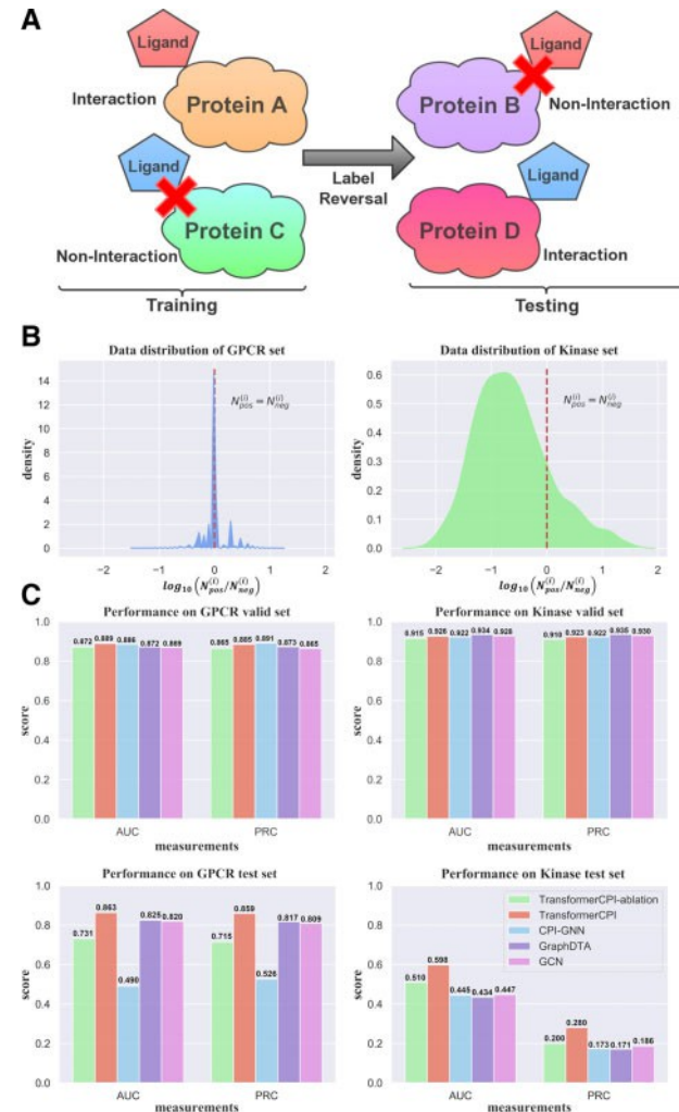
图 3. (A) 标签反转实验示意图: 训练集中的配体只出现在一类样本中 (正作用间 CPI 对或负作用间 CPI 对), 而在测试只出现在另一类样本中。
